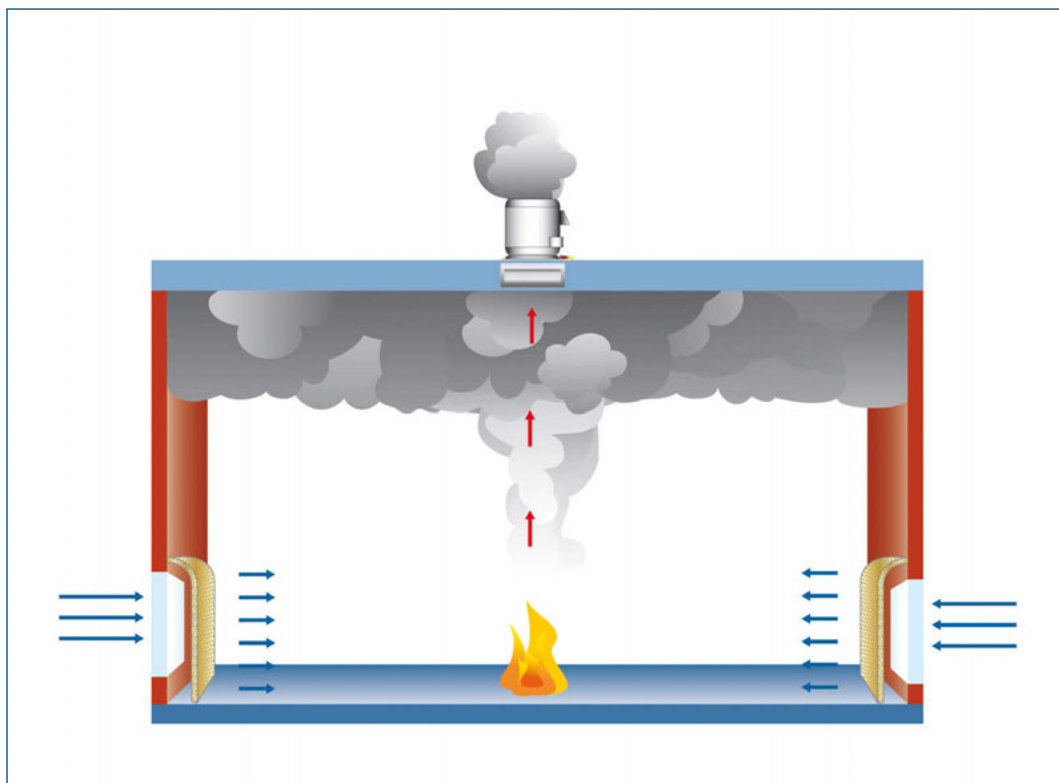
Bild 2: Strömungsgeschwindigkeit der Nachströmung bei Eintritt in den Rauchabschnitt \leq 1 m/s – Reduzierung hoher Nachströmungsgeschwindigkeit, z. B. mit offener, poröser Prallwand
