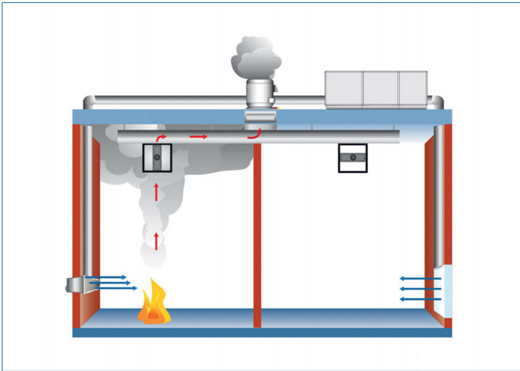
Bild 3: Maschinelle Nachströmung über Quellluftdurchlässe im unteren Raumbereich
