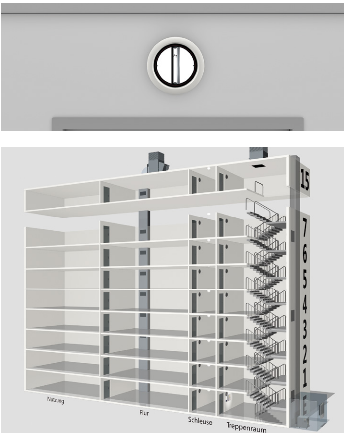
Bild 3: Beispiel einer Rauchschutz-Druck-Anlage – RDA 1
