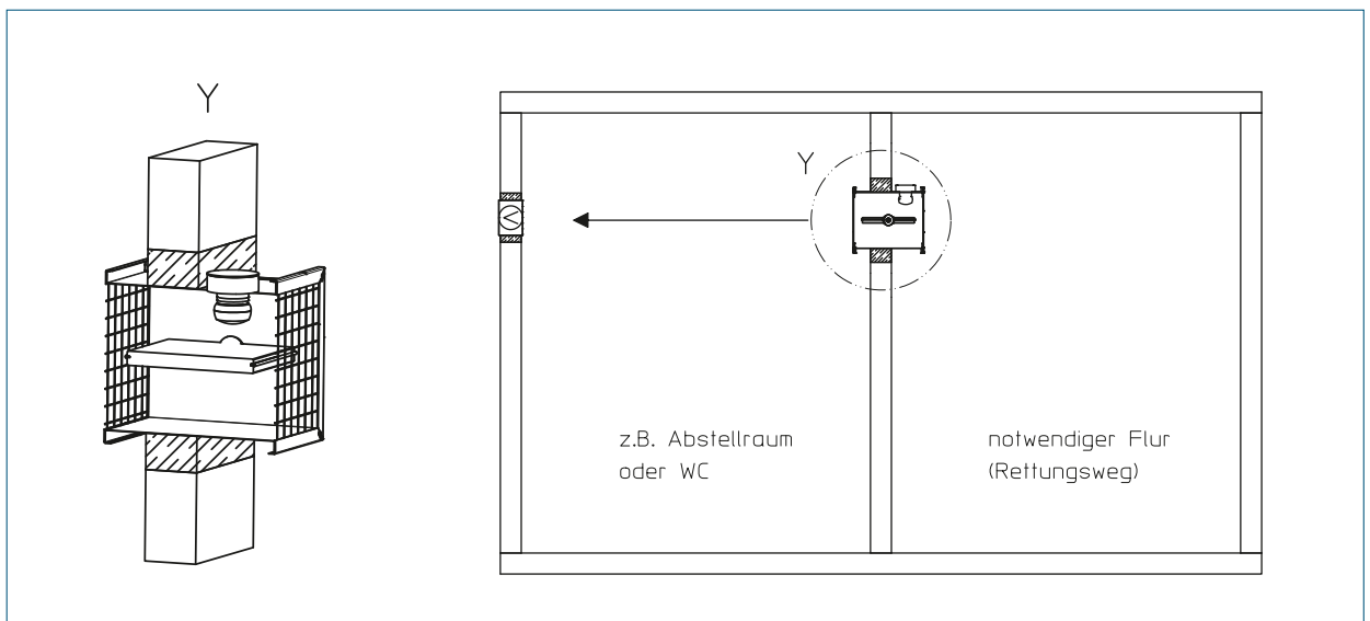
Bild 2: Beispiel eines Bauproduktes nach Z-6.50-... und seiner Anwendung (nicht zu sehen: motorischer Antrieb auf der Rückseite)
