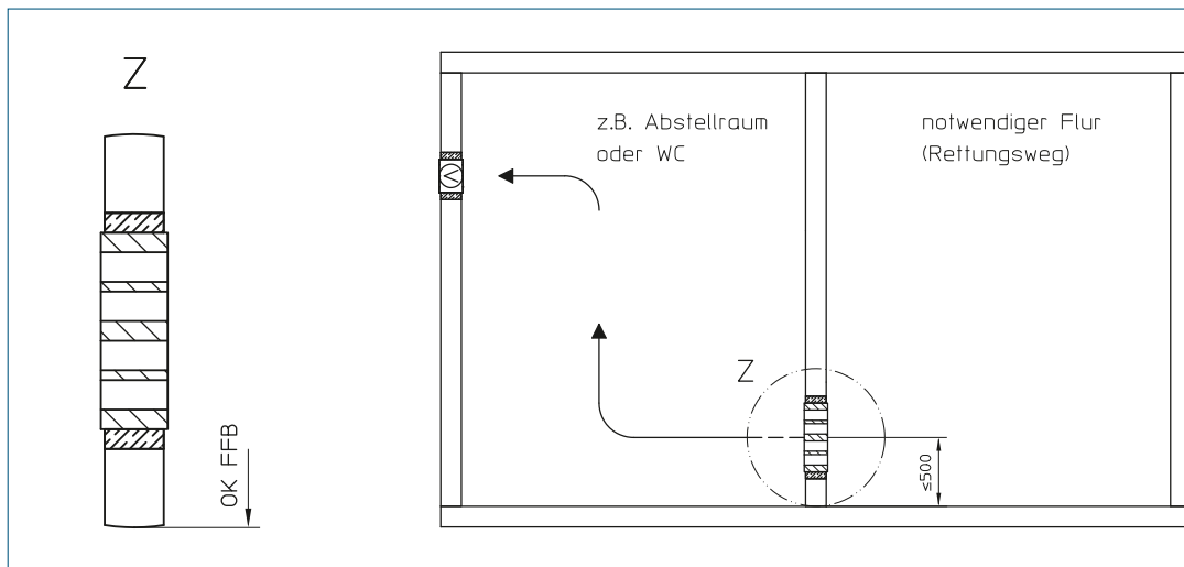
Bild 1: Beispiel eines Bauproduktes nach Z-19.18 und seiner Verwendung
